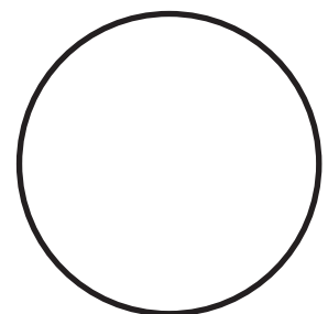
D. Waning Gibbous
